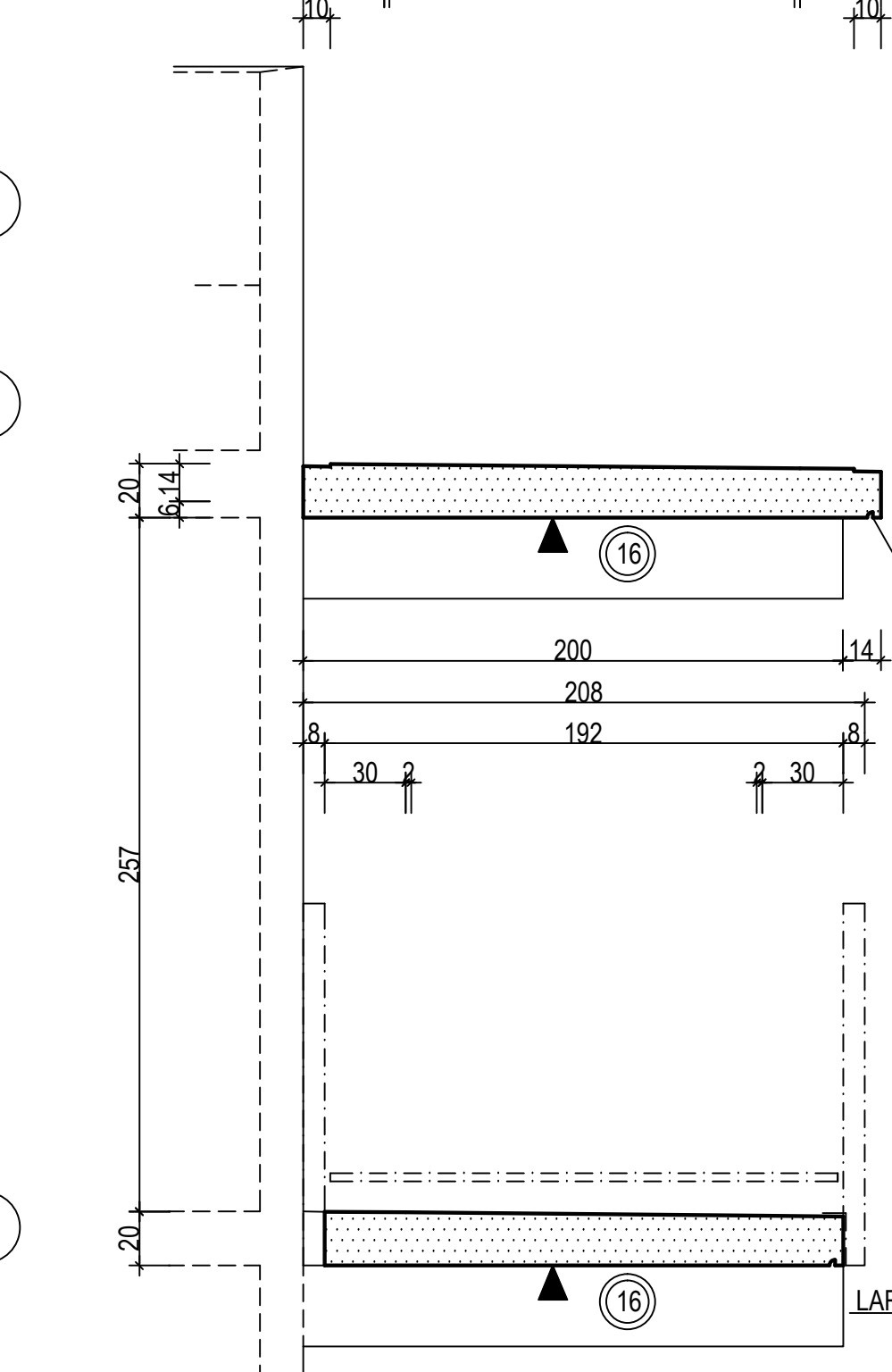
COUPE D Ech: 1/25
