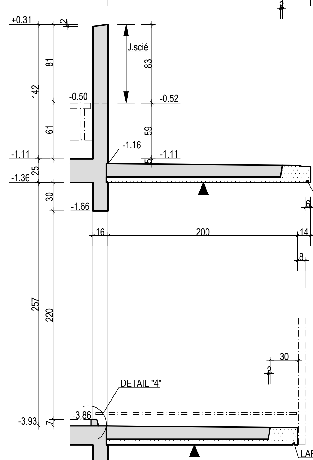
COUPE C Ech: 1/25
