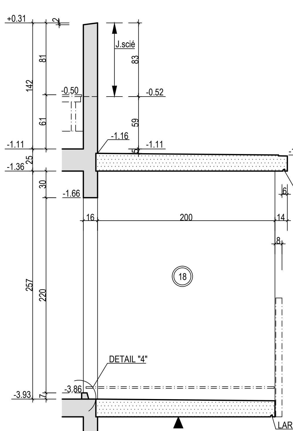
COUPE B Ech: 1/25
