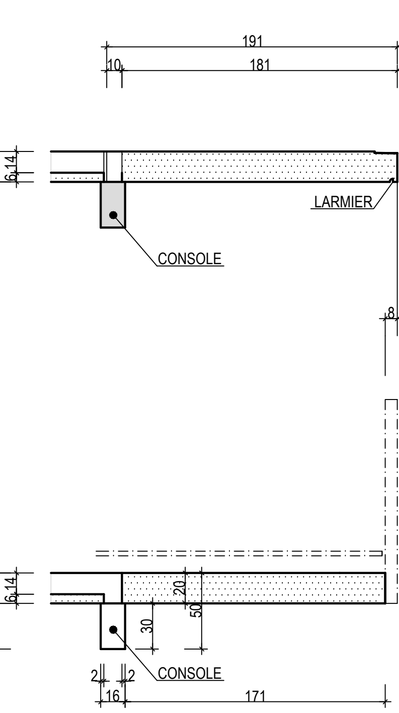
COUPE E Ech: 1/25
