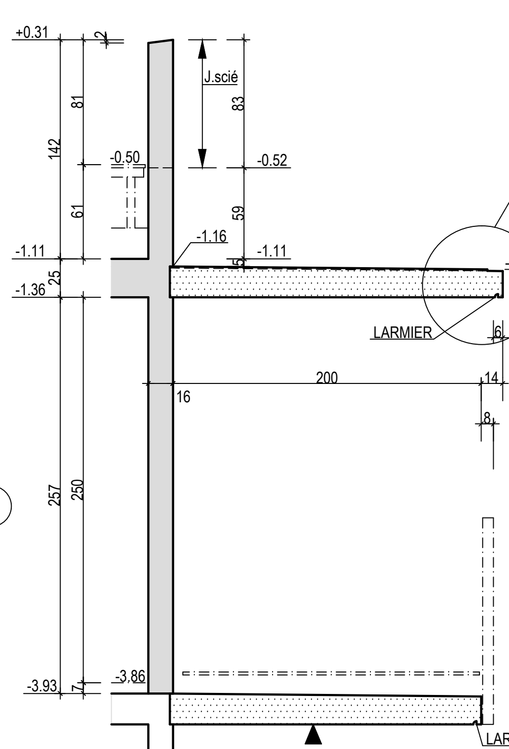
COUPE A Ech: 1/25
